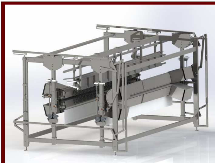
Gerendás kopasztógép
