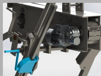
Emelő / állító szerkezet
