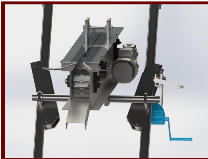
Fej és légcső eltávolító gép
